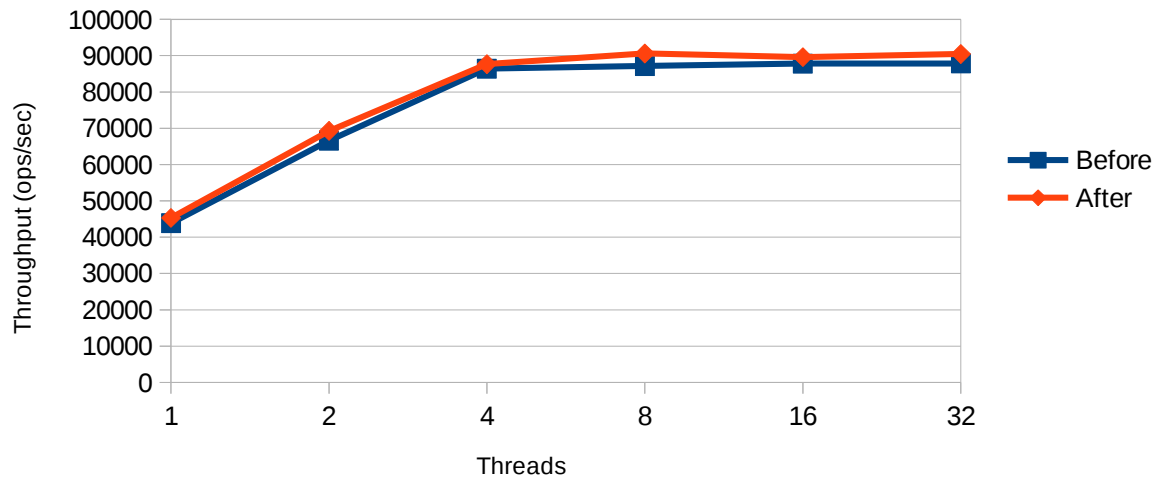
Policy.getPermissions(CodeSource)
